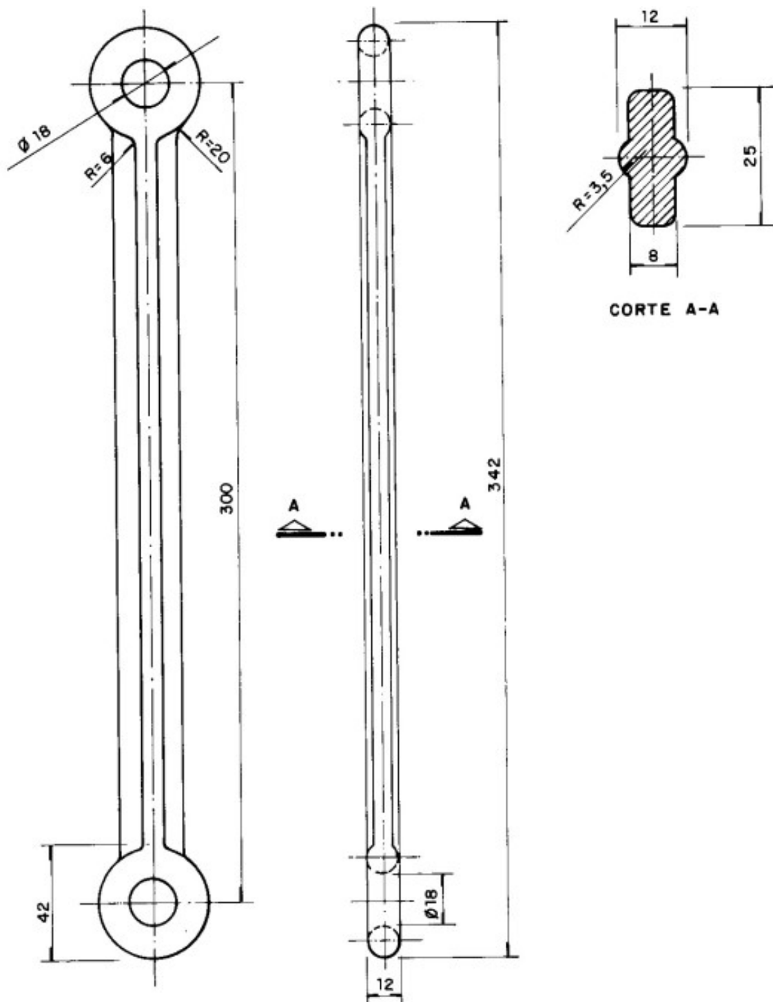
Figura 1 – Prolongador Olhal-Olhal
